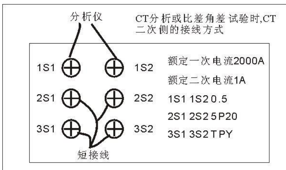
图 3.4.1 CT 分析和比差角差试验时，CT 二次侧参考接线图
