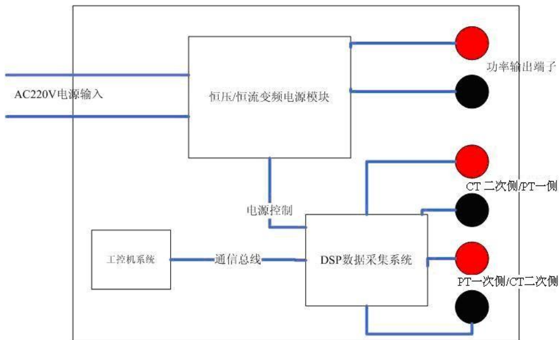
图 2.3 CT 分析仪硬件原理图
