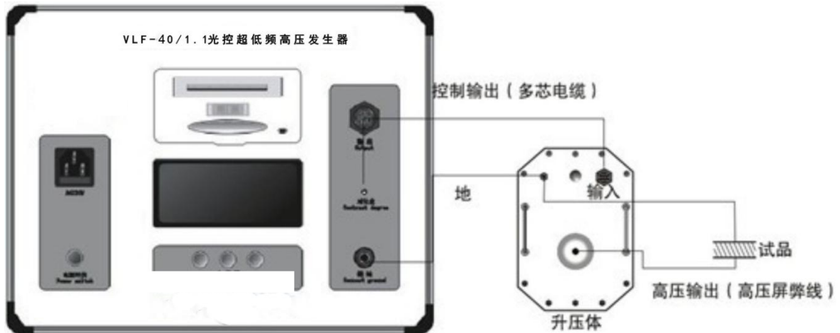
图 4a VLF-40/1.1 或 VLF-50/1.1 (连接图)
