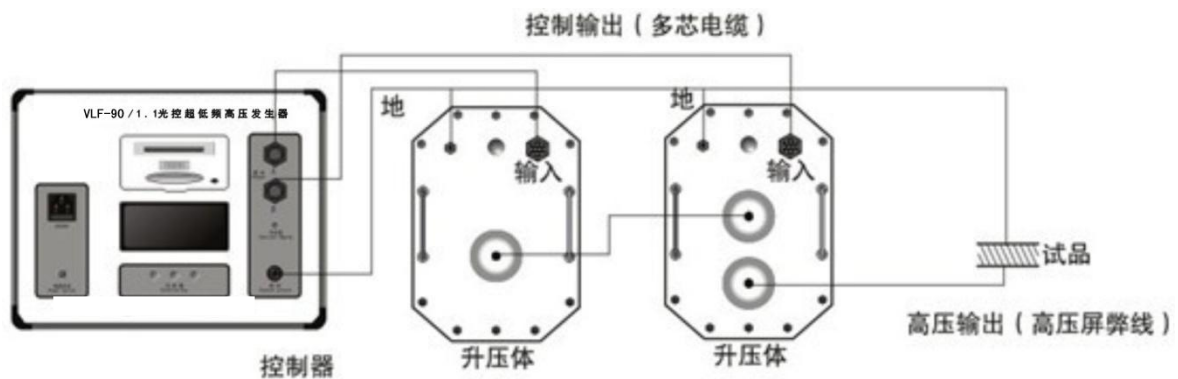
图 4b VLF-90/1.1 (连线图)
