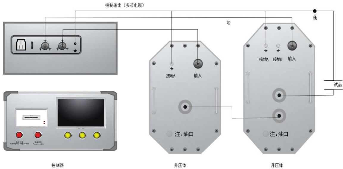
图 4b VLF-80/1.1 (连线图)
