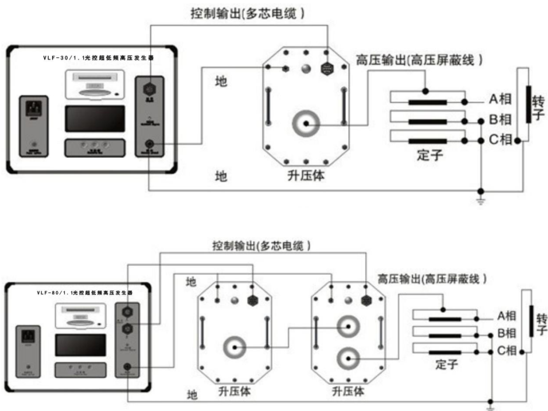
图18a/b 测量定子的某相连线图
