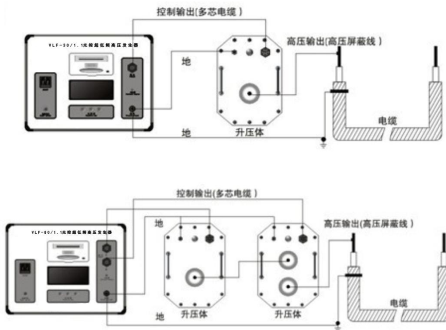
图17a/b 单相测量连线图
