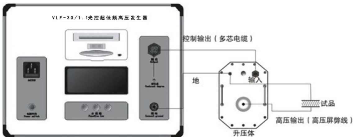
图 4a VLF-30/1.1 或 VLF-50/1.1 (连接图)
