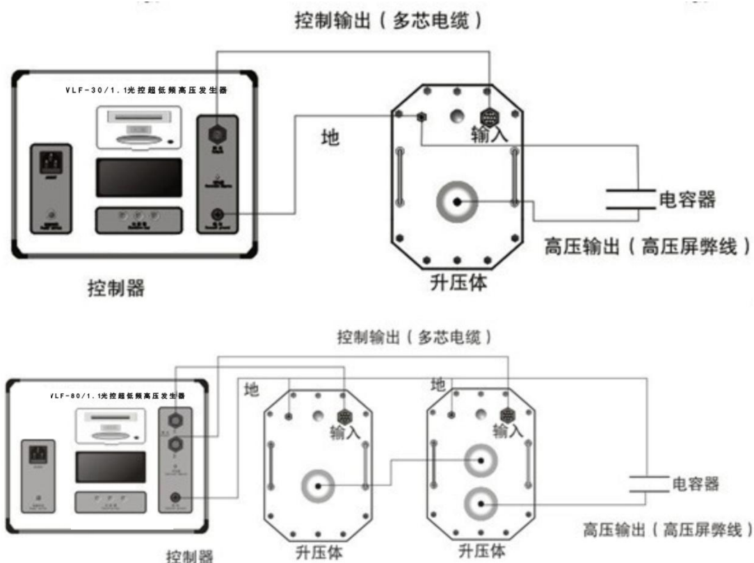
图19a/b 测量电容器的连线图
